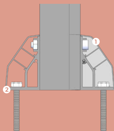
Assemblage de la clôture
