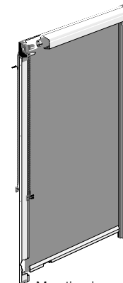
Moustiquaire enroulable pour porte "Moustiroll". Manoeuvre à double chaînette
